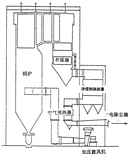
图 3.1-8 包含氨催化剂接触还原脱硫装置 的整体配置图
